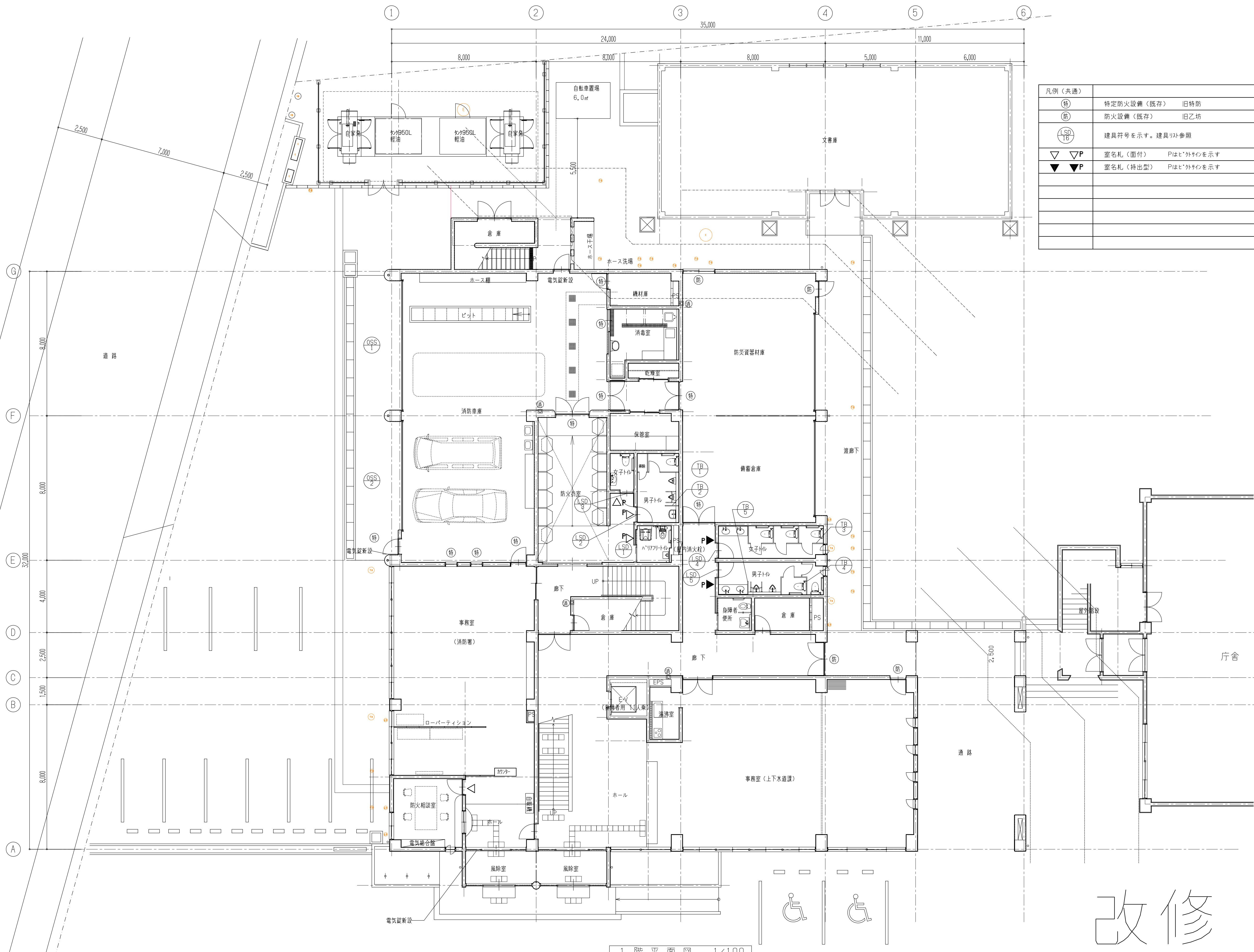
1 階 平 面 図 1/100
