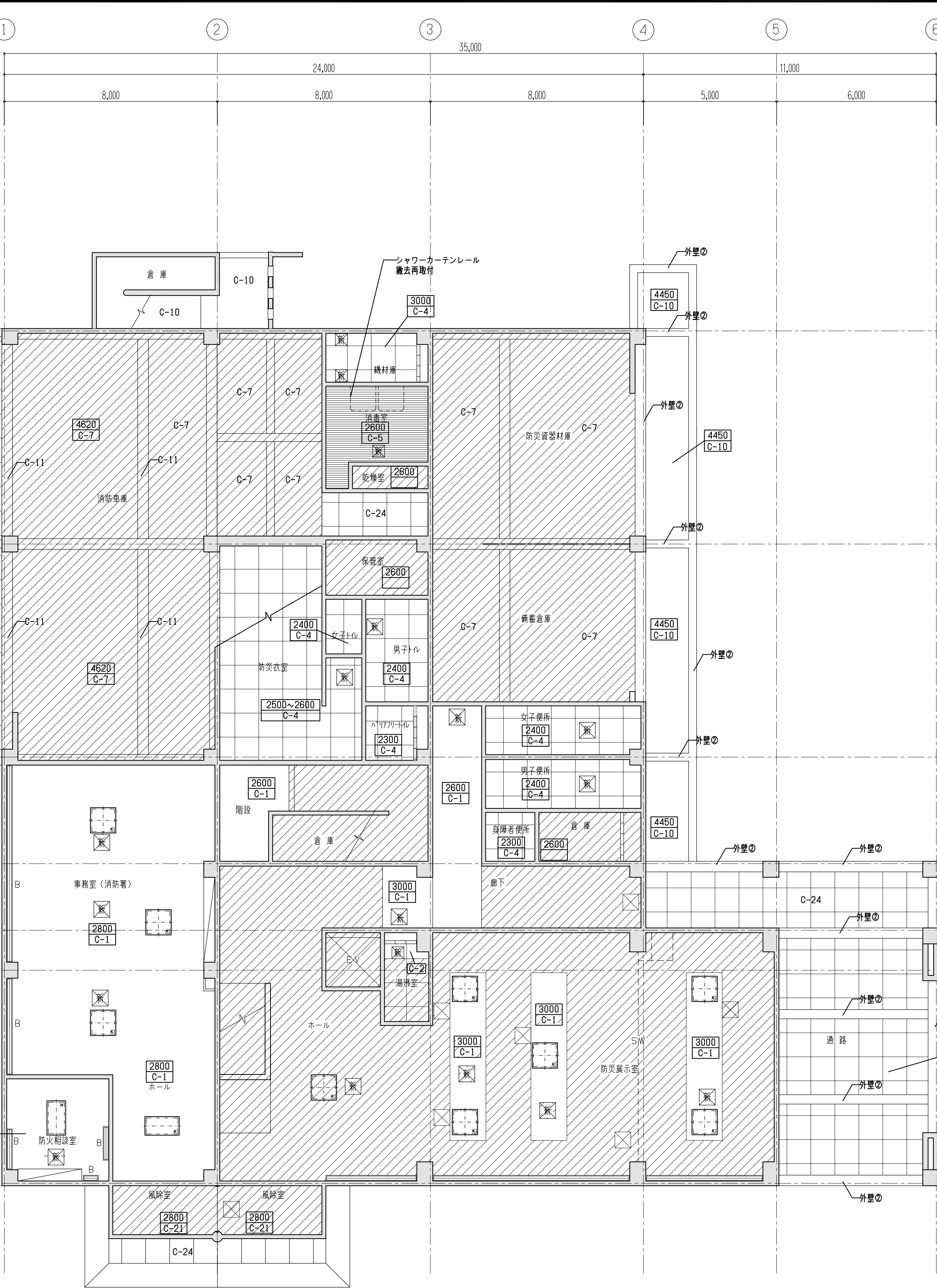
1 階 天 井 伏 図 1/100
