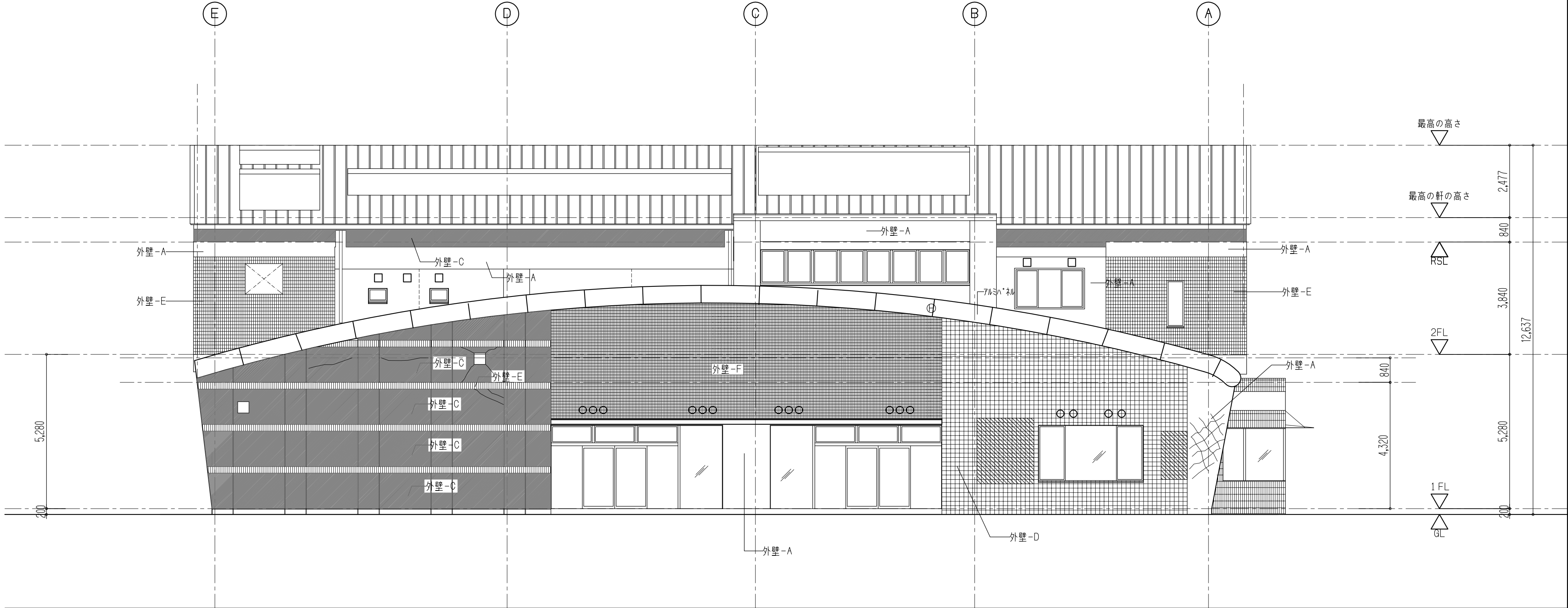
西側立面図 1/100
