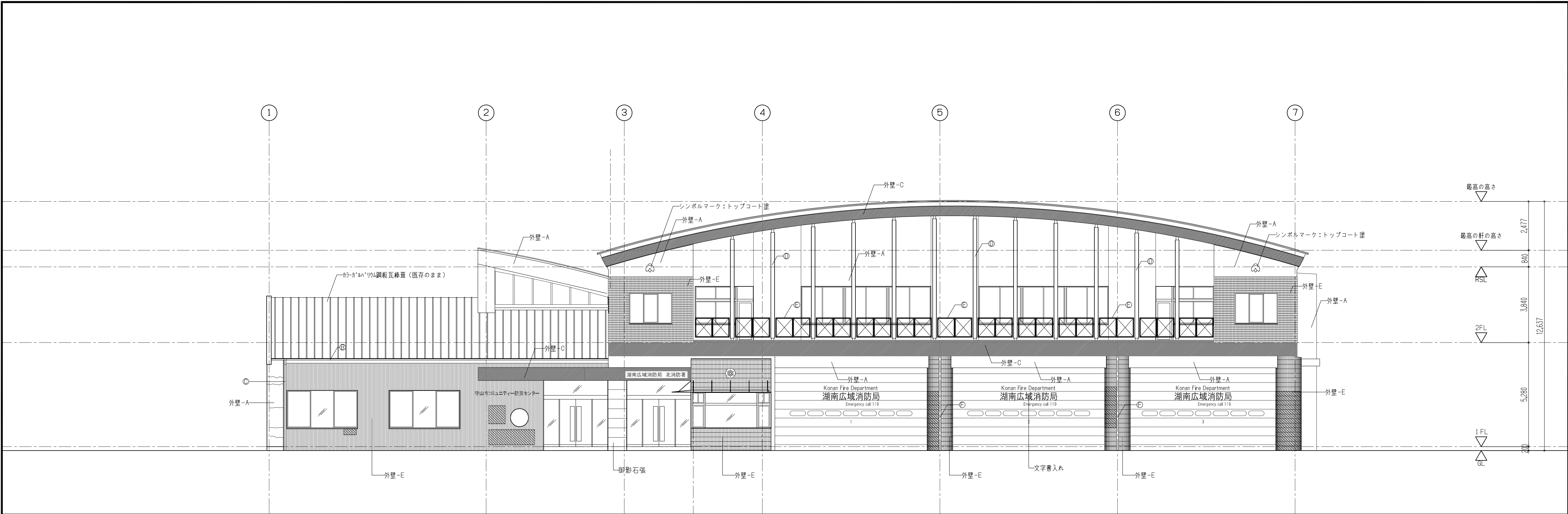
南側立面図 1/100
